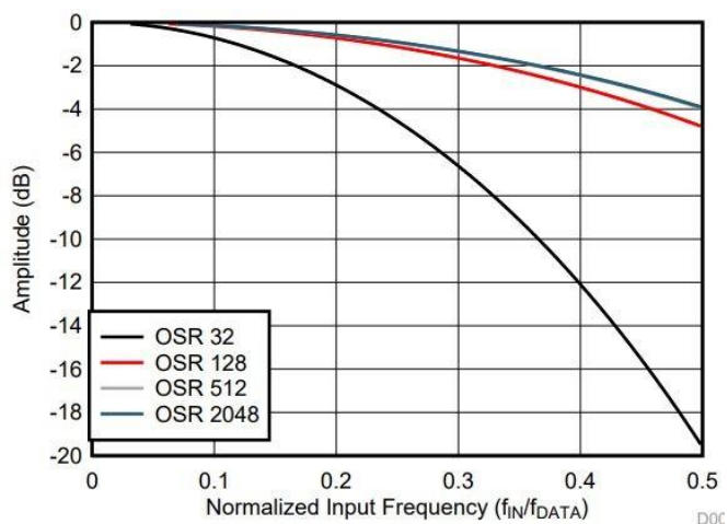
Figure 4 : Fonction de transfert du filtre Low Latency pour des fréquences inférieures à la limite de Shannon
