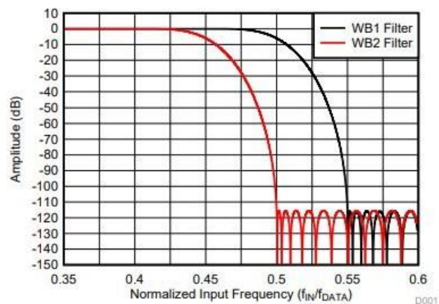
Figure 3 : Comparaison des fonctions de transfert des filtres WB1 et WB2
