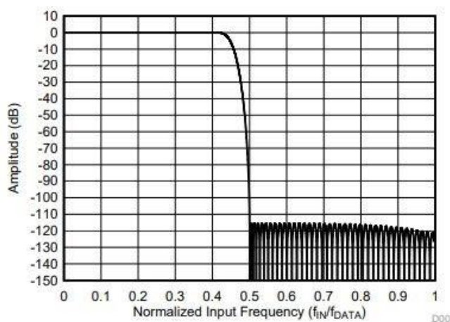
Figure 2 : Fonction de transfert du filtre WB2
